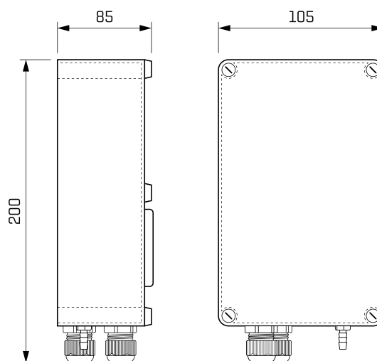
Rys. 1: Wymiary urządzenia w mm
