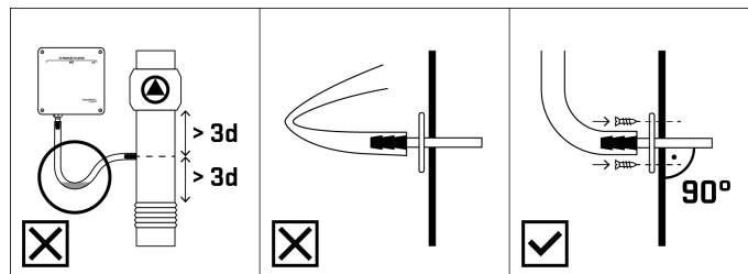
Rys. 3: Zalecenia montażowe
